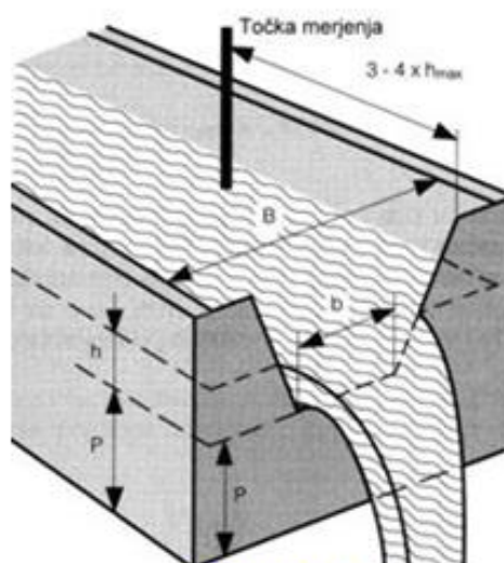
Trapezoidni jez.
