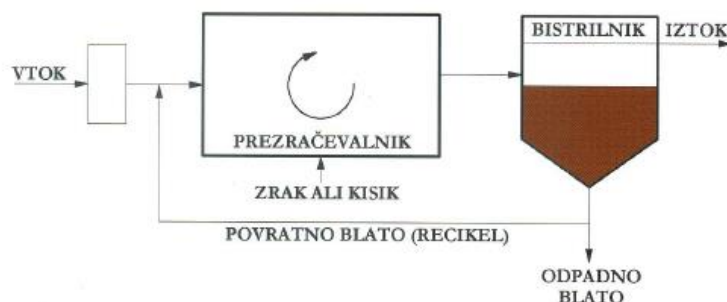
Slika 45: Shema sistema s popolnoma premešanim reaktorjem aktivnega blata s "selektorjem" Vir: Roš in Zupančič, 2010, 112
